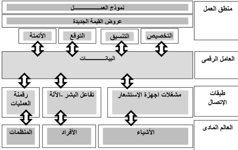
الشكل 11.3 إطار الكثافة الرقمية
